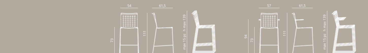
Sgabello con o senza braccioli / Stool with or without arms
