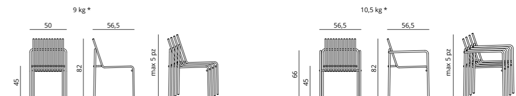
Sedia con e senza braccioli / Chair with and without arms
