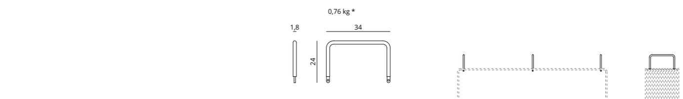
Bracciolo panca piana / Armrest flat bench
