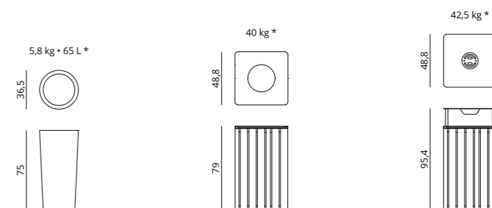
Contenitore interno + cestone + cestone accessoriabile / Inner container + big litter bin + customizable big litter bin
