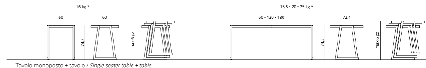
Tavolo monoposto + tavolo / Single-seater table + table
