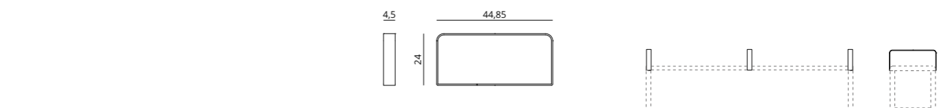
Bracciolo panca piana / Armrest flat bench
